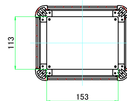
C-C ( 1 : 5 )
