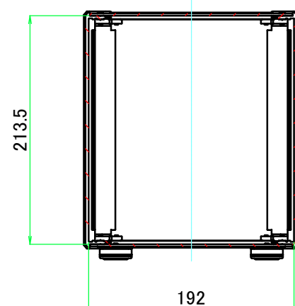
A-A ( 1 : 5 )
